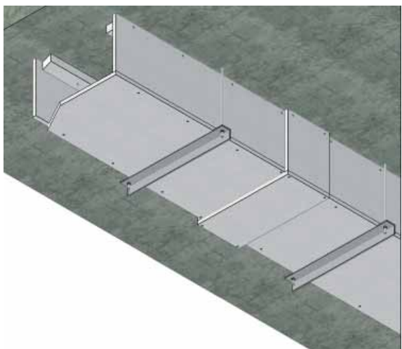
1. Conducto horizontal 3 caras.
